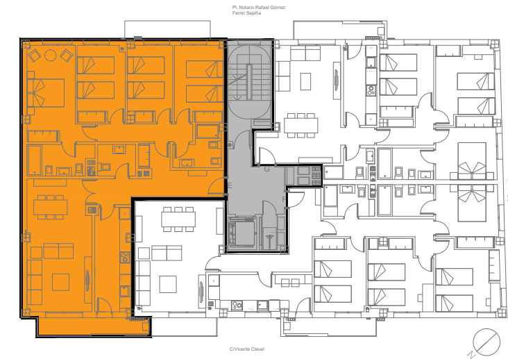
PLANTAS 4ª, 5ª, 6ª y 7ª. VIVIENDA TIPO - E
